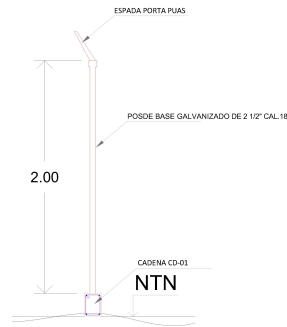
SECCIÓN TRANSVERSAL
