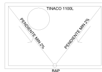
PLANTA DE AZOTEA
