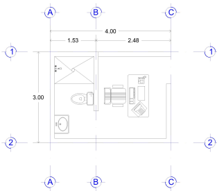
PLANTA ARQUITECTÓNICA
