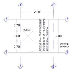
ACERO LONGITUDINAL
