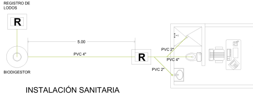
INSTALACIÓN SANITARIA
