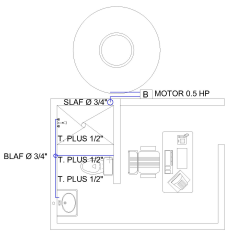
INSTALACIÓN HIDRÁULICA
