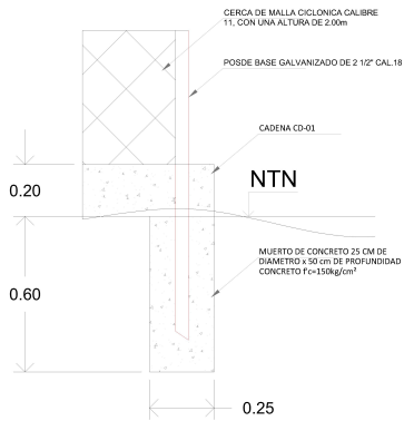
DETALLE DE CIMENTACIÓN
