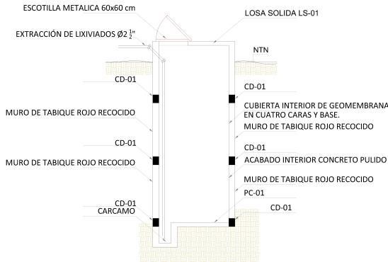
CARCAMO EN ALZADO
