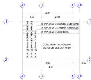
LOSA DE AZOTEA
