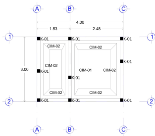
PLANTA DE CIMENTACIÓN
