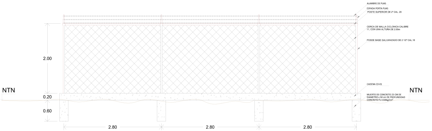
CERCA PERIMETRAL
