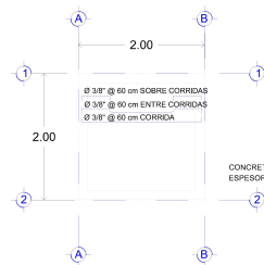
ACERO TRANSVERSAL
