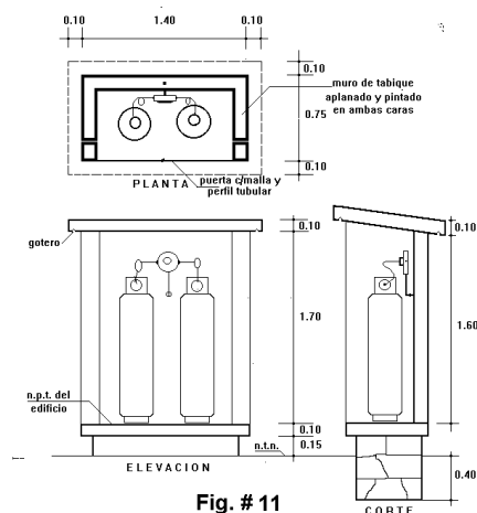
Fig. # 11 CASETA PARA TANQUES DE GAS
