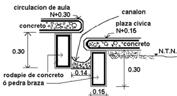
DETALLE PARA CAMBIO DE NIVEL
