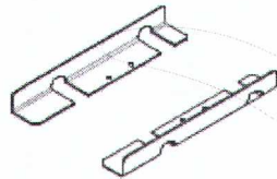
DETALLE DE PIEZA DE LAMINA PARA UNIR ASNILLAS Y ASIENTO
