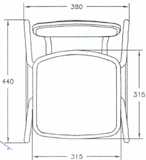
VISTA SUPERIOR
