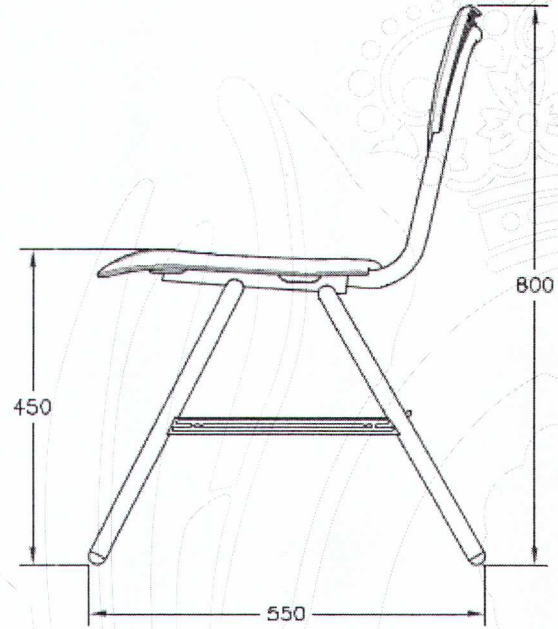
VISTA LATERAL
