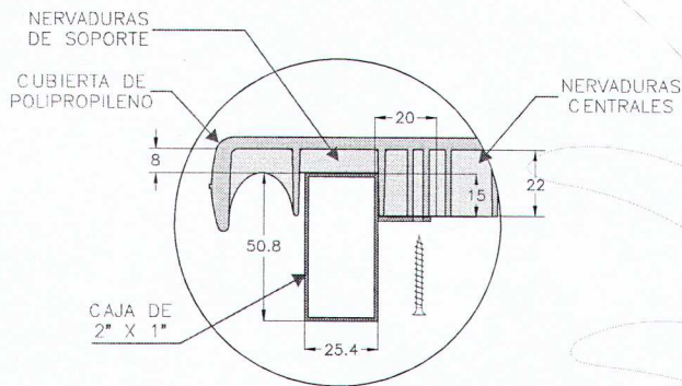
DETALLE DE UNIÓN DE LA CUBIERTA CON LA ESTRUCTURA
