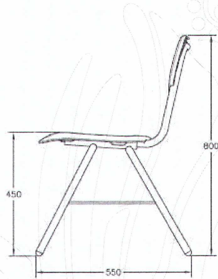
VISTA LATERAL
