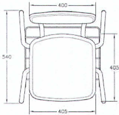
VISTA SUPERIOR
