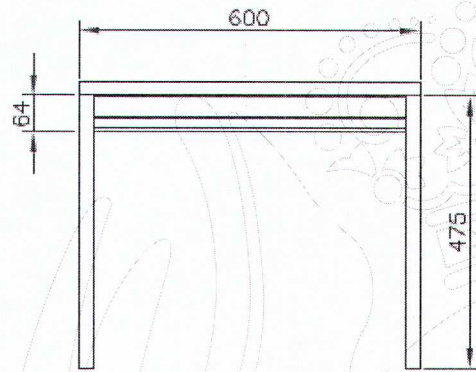
VISTA LATERAL
