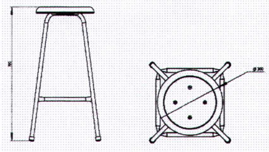
BANCO PARA SENTARSE
