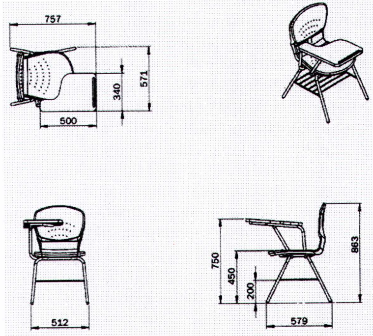
SILLA DE PALETA
