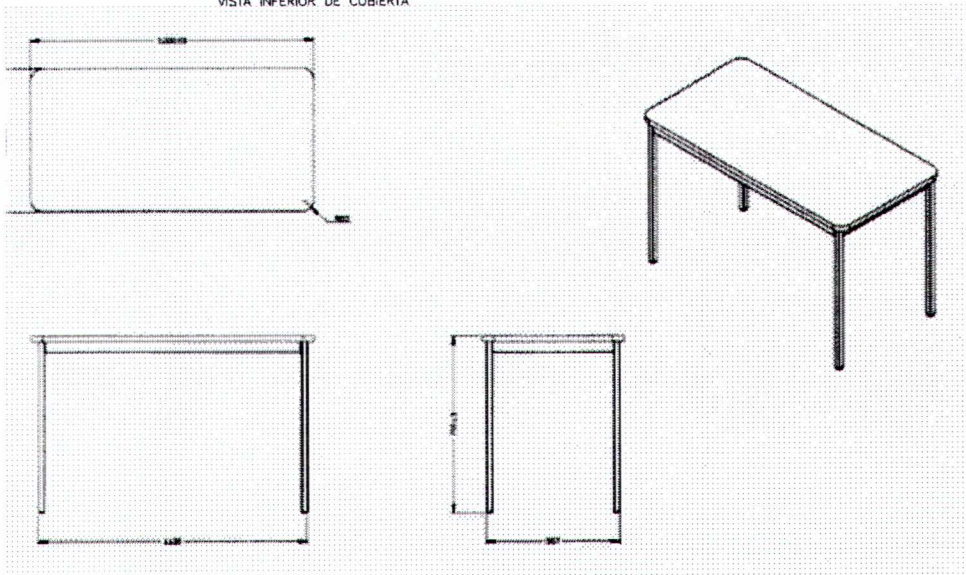
VISTA INFERIOR DE CUBIERTA
