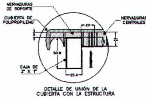
DETALLE DE UNIÓN DE LA CUBIERTA CON LA ESTRUCTURA
