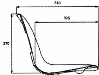
VISTA LATERAL EN CORTE ASIENTO RESPALDO
